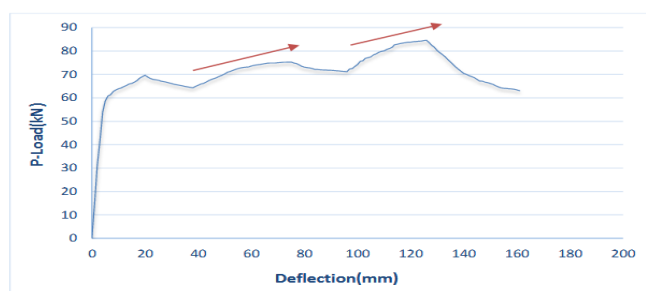
شکل ۲؛ اثر پدیده سخت‌شوندگی ناشی از پل زدن الیاف‌ها را در نمونه‌های ۳٪ الیاف B-H-۴ ، B-H-۳
