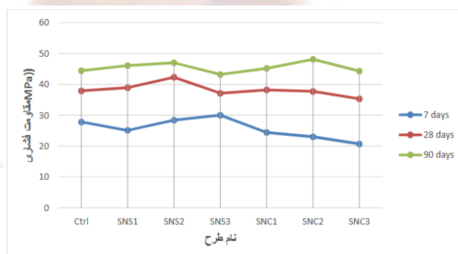
نمودار ۷؛ بررسی تغییرات مقاومت فشاری در سنین مختلف نمونه‌های نانو
