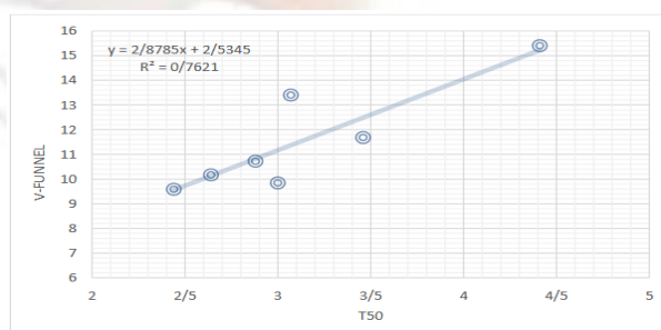
نمودار ۴: ارتباط بین زمان قیف V و T_{50} در مخلوط‌های با درصد‌های مختلف نانو
