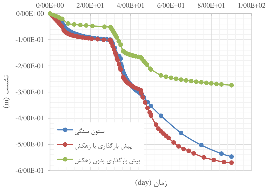
شکل ۳: مقایسه نشست های ناشی از بارگذاری سربار به سه حالت حضور ستون های سنگی، حضور و عدم حضور زهکش های شعاعی
