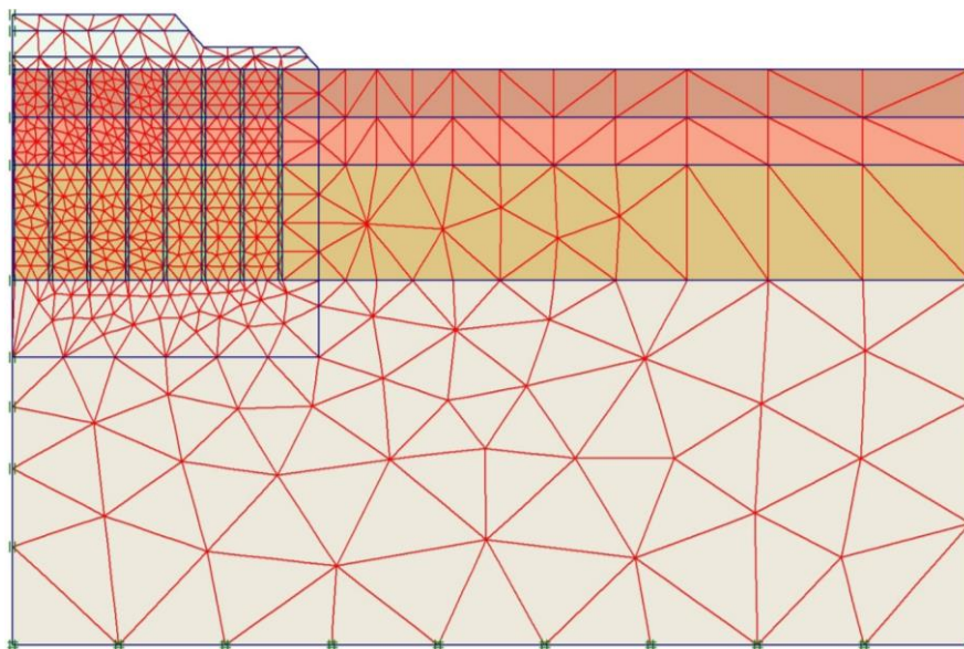
شکل ۱: هندسه و المان بندی مدل ستون سنگی
