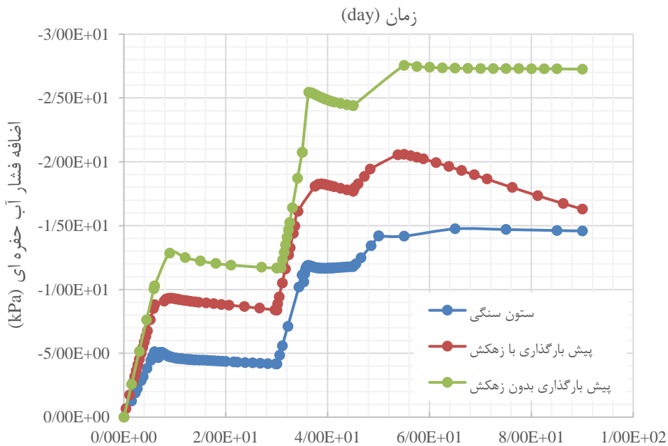
شکل ۴: مقایسه فشار آب حفره ای اضافی ناشی از بارگذاری سربار به سه حالت حضور ستون های سنگی، حضور و عدم حضور زهکش های شعاعی
