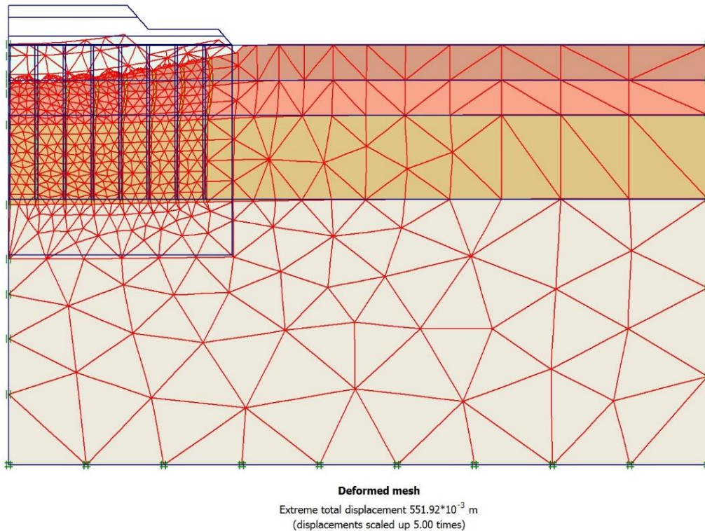
شکل ۲: تغییر شکل مدل ستون سنگی در ساختمانی مدل پیش بارگذاری
