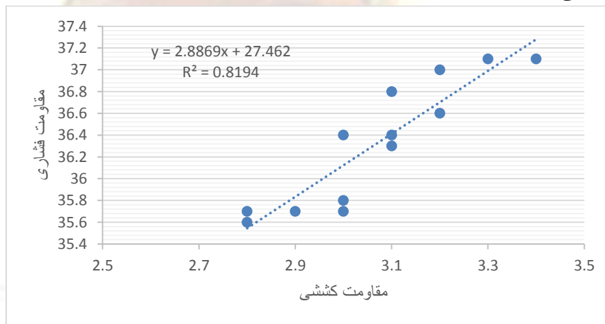
شکل ۱۵: تغییرات مقاومت کششی با مقاومت فشاری در بتن‌های حاوی درصدی متفاوت PET.
