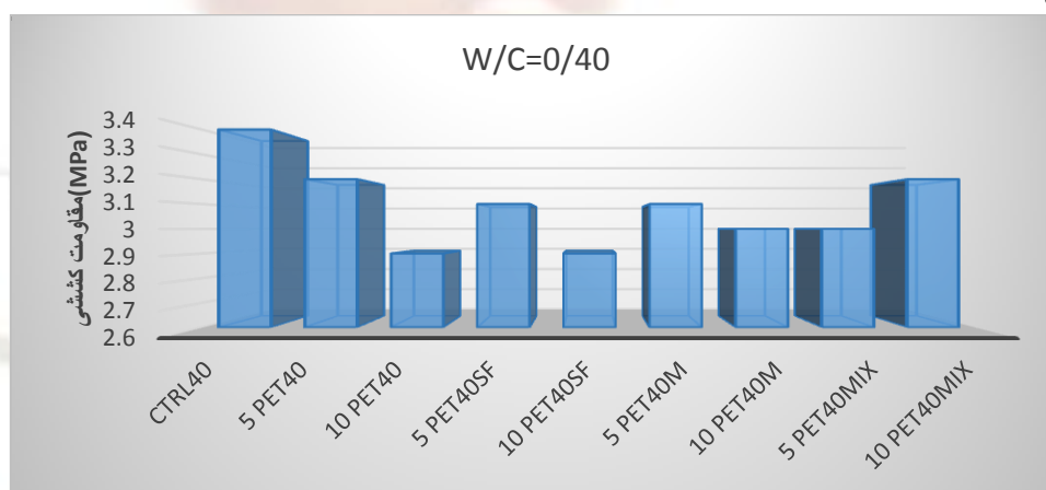
شکل ۱۱: تغییرات مقاومت کششی با گذشت زمان برای بتن با نسبت (W/C=0.4) و درصدهای مختلف PET.
