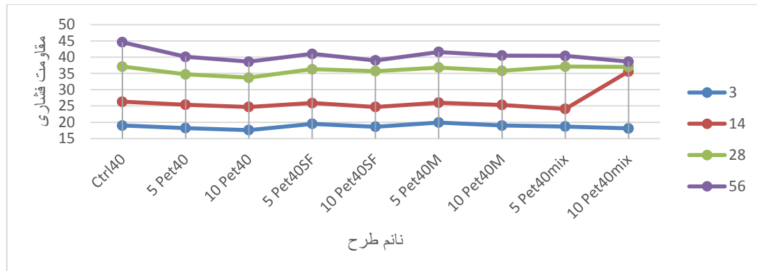
شکل ۹: تغییرات فشاری باگذشت زمان برای بتن با (W/C=۰/۴۰) و درصدهای مختلف PET.
