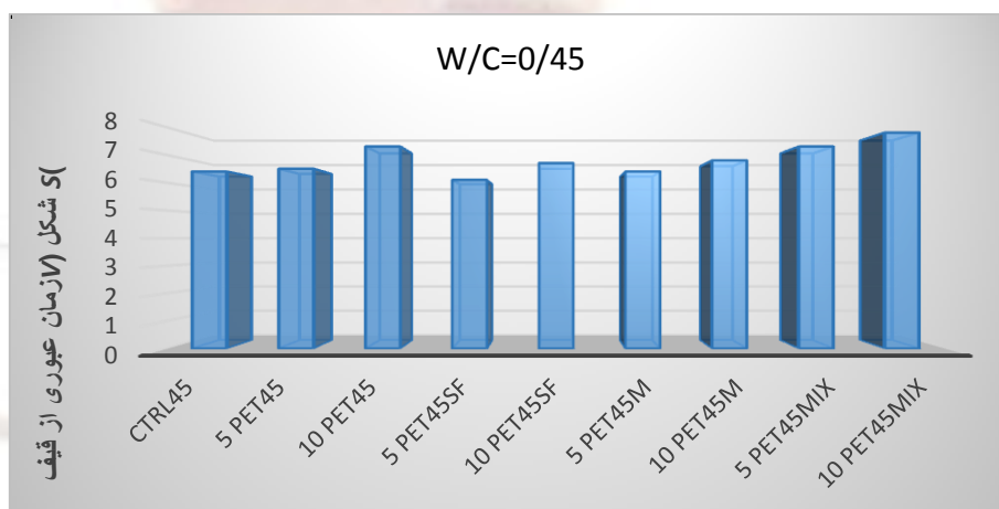
شکل ۴: آزمایش قیف V شکل به ازای درصدهای مختلف PET برای نسبت آب به سیمان ۰/۴۵.
