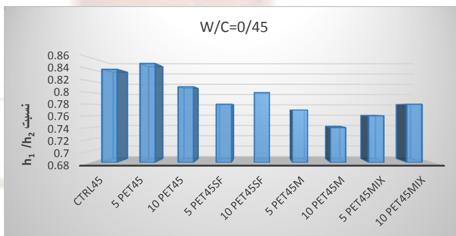
شکل ۶: نسبت h_1/h_2 به ازای درصدهای مختلف PET برای نسبت آب به سیمان ۰/۴۵.
