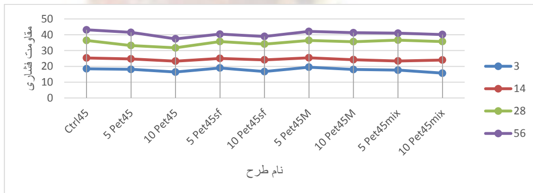
شکل ۱۰: تغییرات فشاری باگذشت زمان برای بتن با (W/C=۰/۴۵) و درصدهای مختلف PET.
