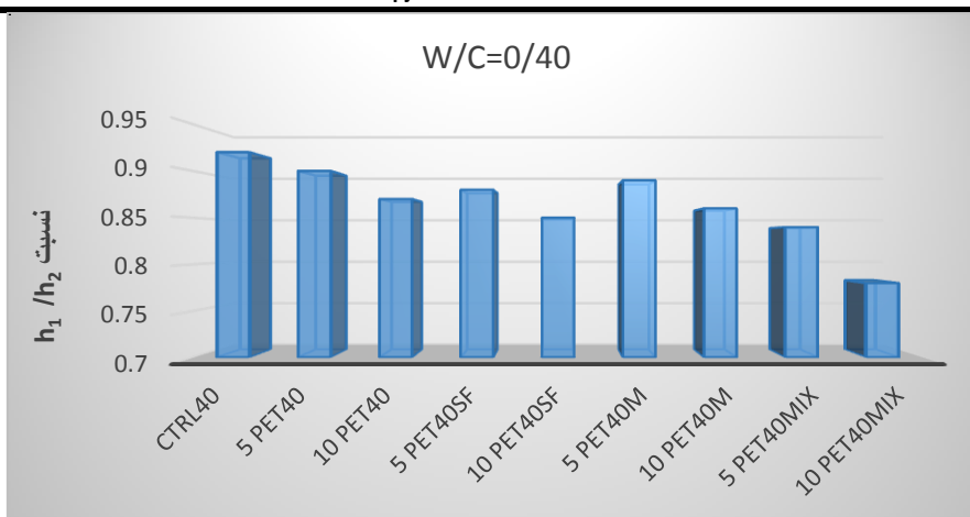
شکل ۵: نسبت h_1/h_2 به ازای درصدهای مختلف PET برای نسبت آب به سیمان ۰/۴۰.
