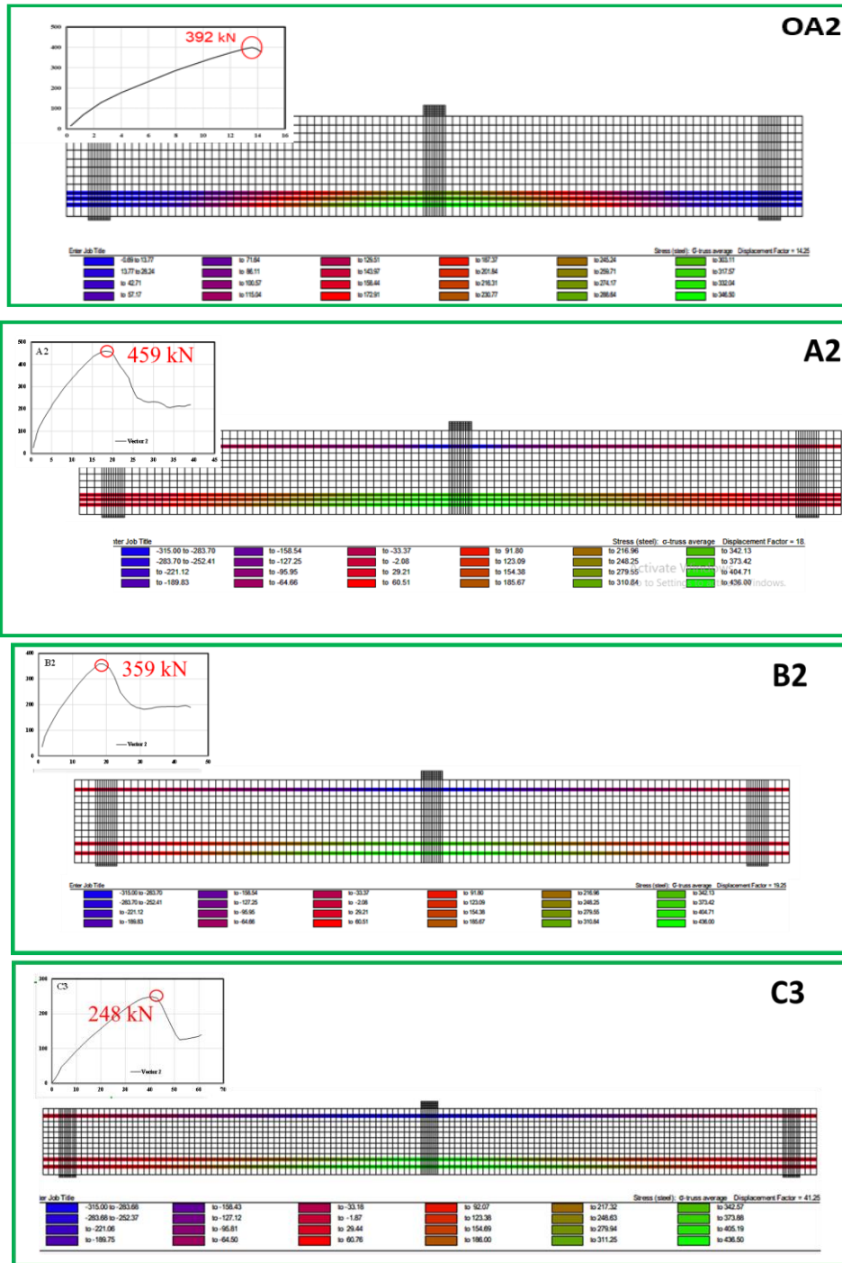
شکل 8 توزیع تنش در میلگردهای تیرهای بتن مسلح
