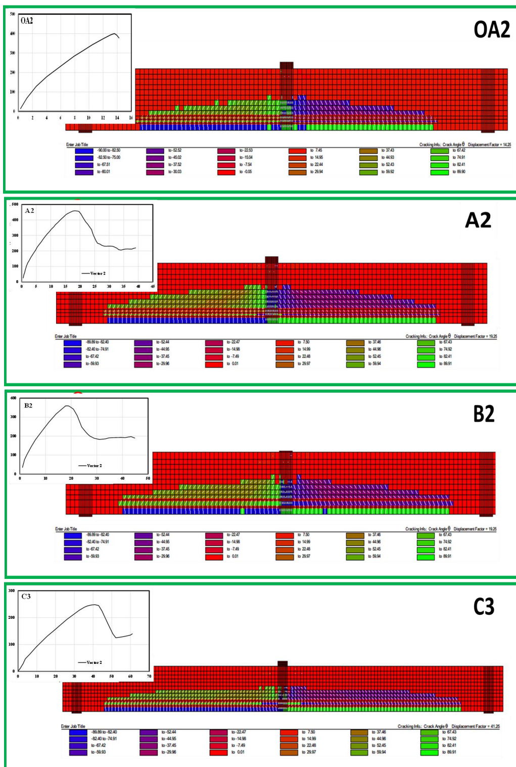
شکل 9 ترکیب جابه جایی و ترک خوردگی
