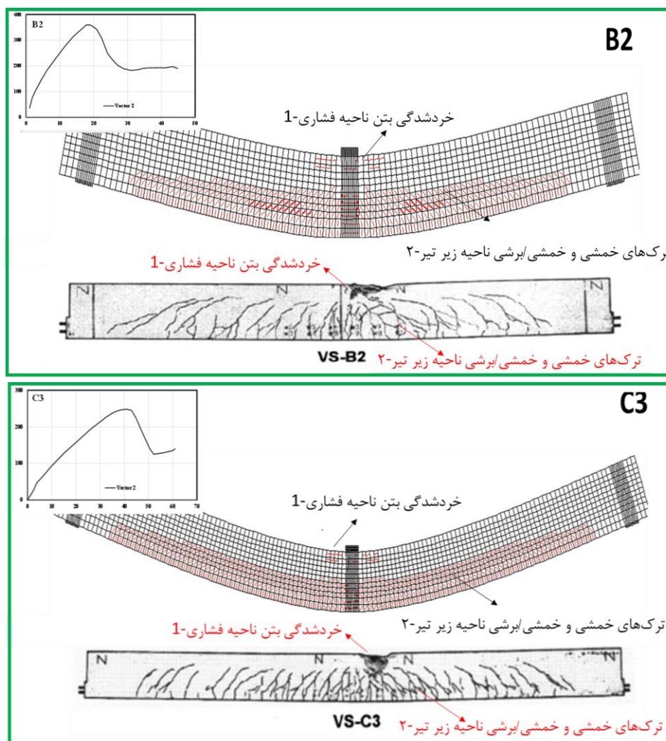
شکل 10 مقایسه توزیع ترک خوردگی بین حالت آزمایشگاهی [14] و نرم افزار Vector 2.
