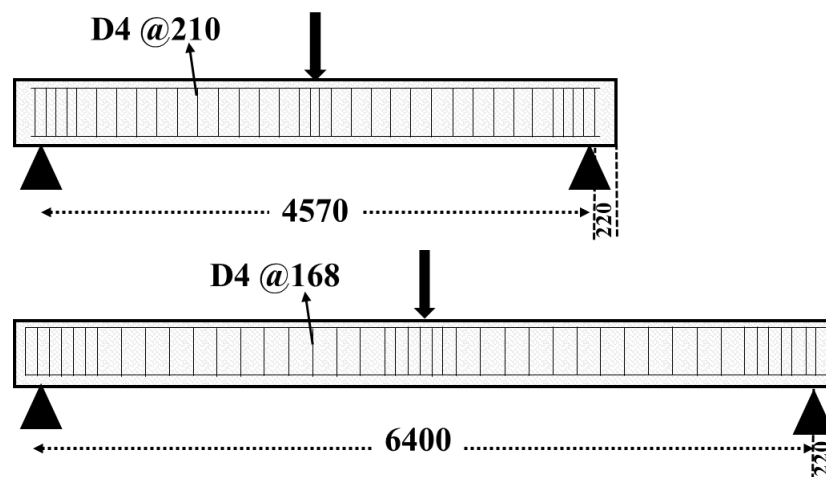
شکل 3 مقطع طولی تیرهای [14]
