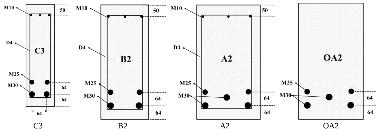
شکل 2 مقطع عرضی تیرهای بتنی [14]
